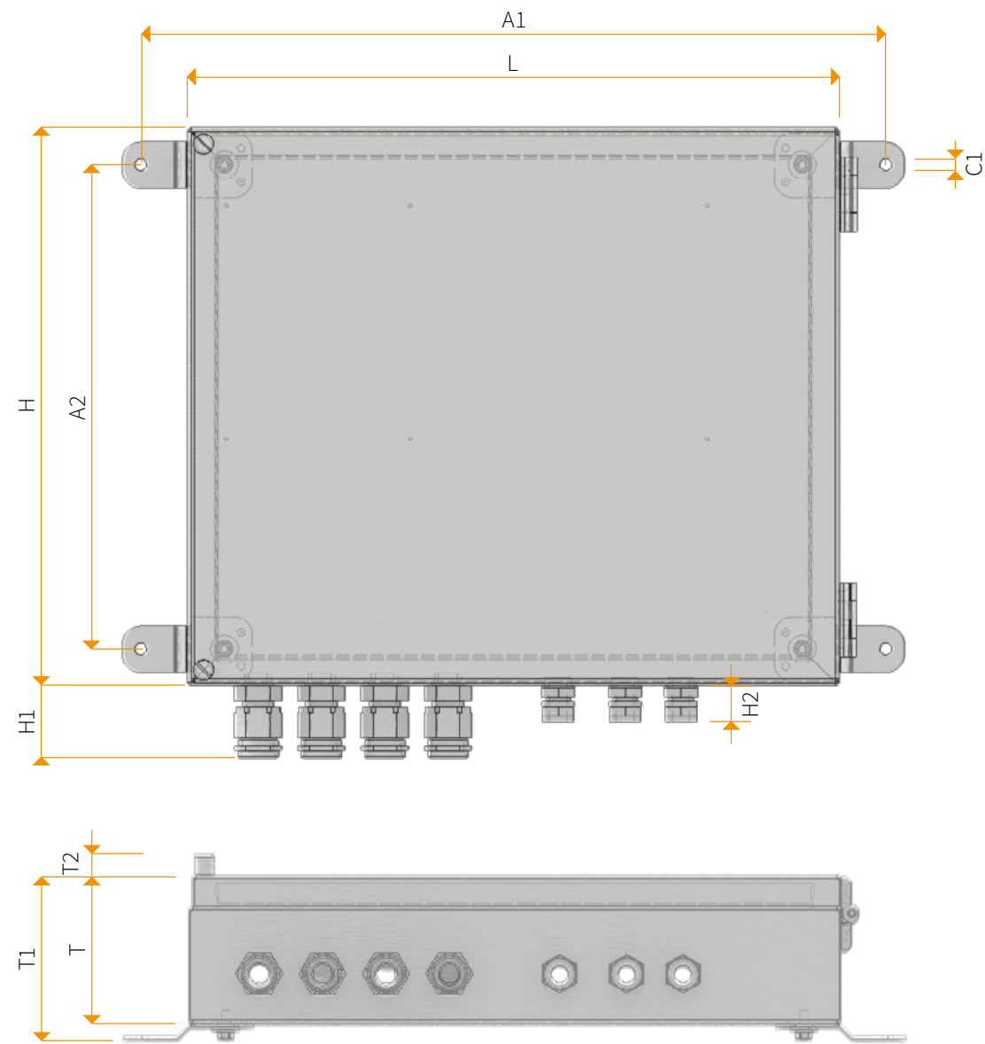
Abbildung 2: Standard-Abmessungen des EdgerKraft Controllers (MMV)
