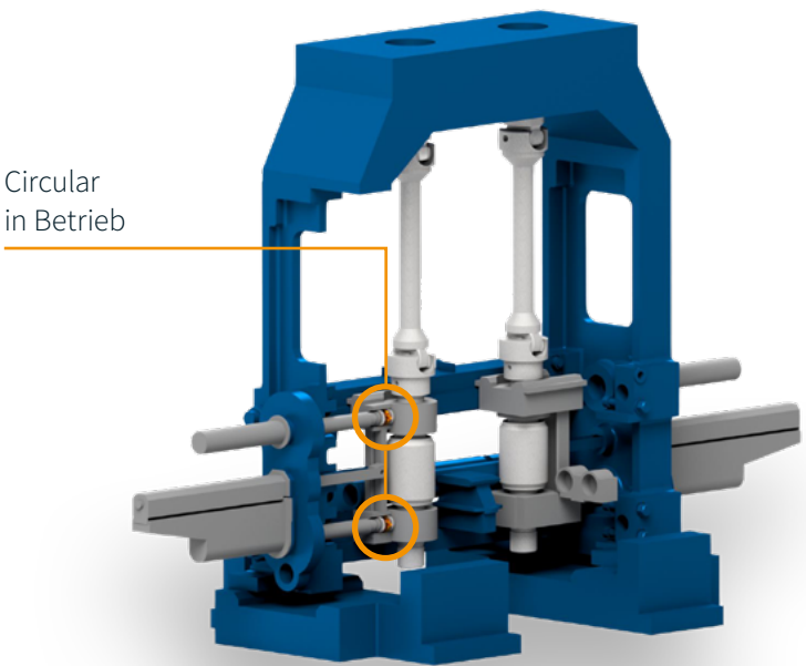
Abbildung 1: Illustration einer vertikalen Stauchpresse, die mit EdgerKraft Circular ausgestattet ist
