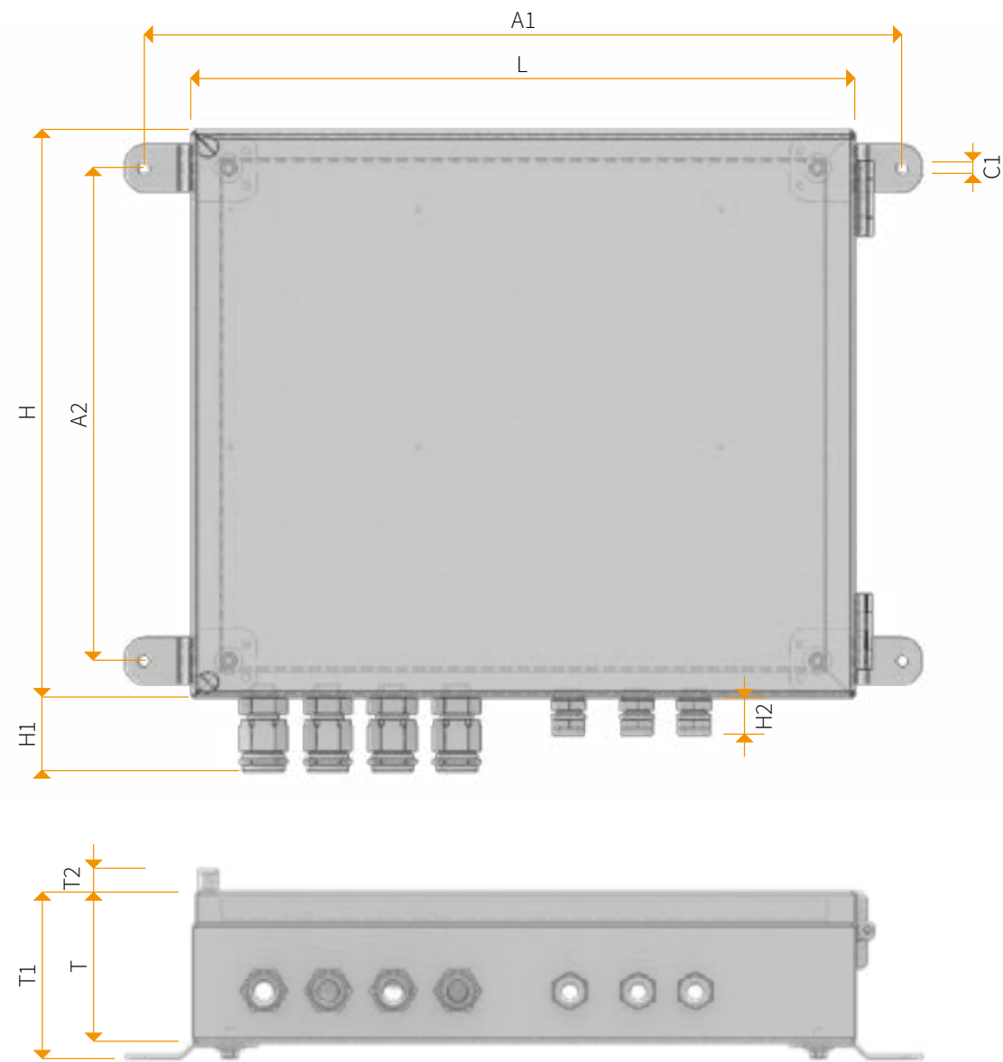
Abbildung 2: Standard-Abmessungen des RollKraft Controllers (MMV)
